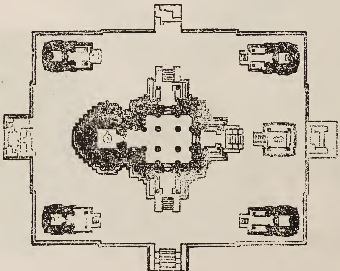
Fig. 30 Sinnar, Gondesvara temple: Plan
