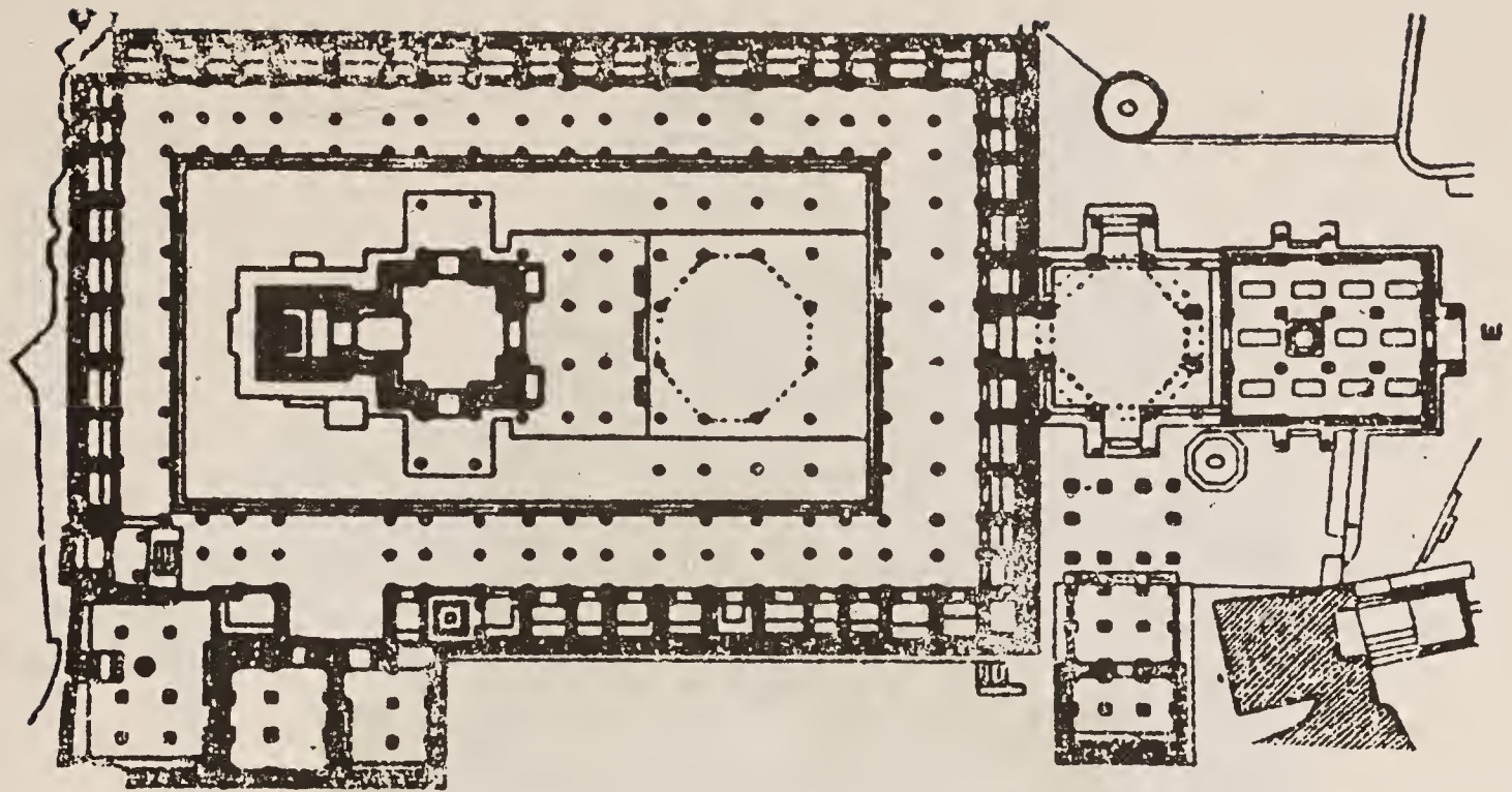
Fig. 12 Dilwārā, Vimala's temple: Plan
