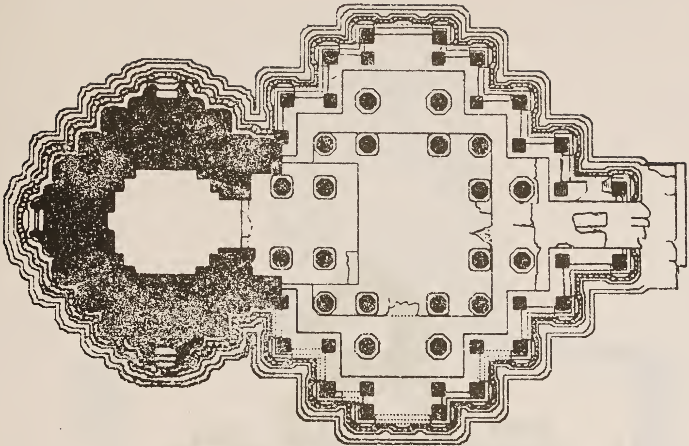
Fig. 21 Sejakpur, Navalākhā temple: Plan
