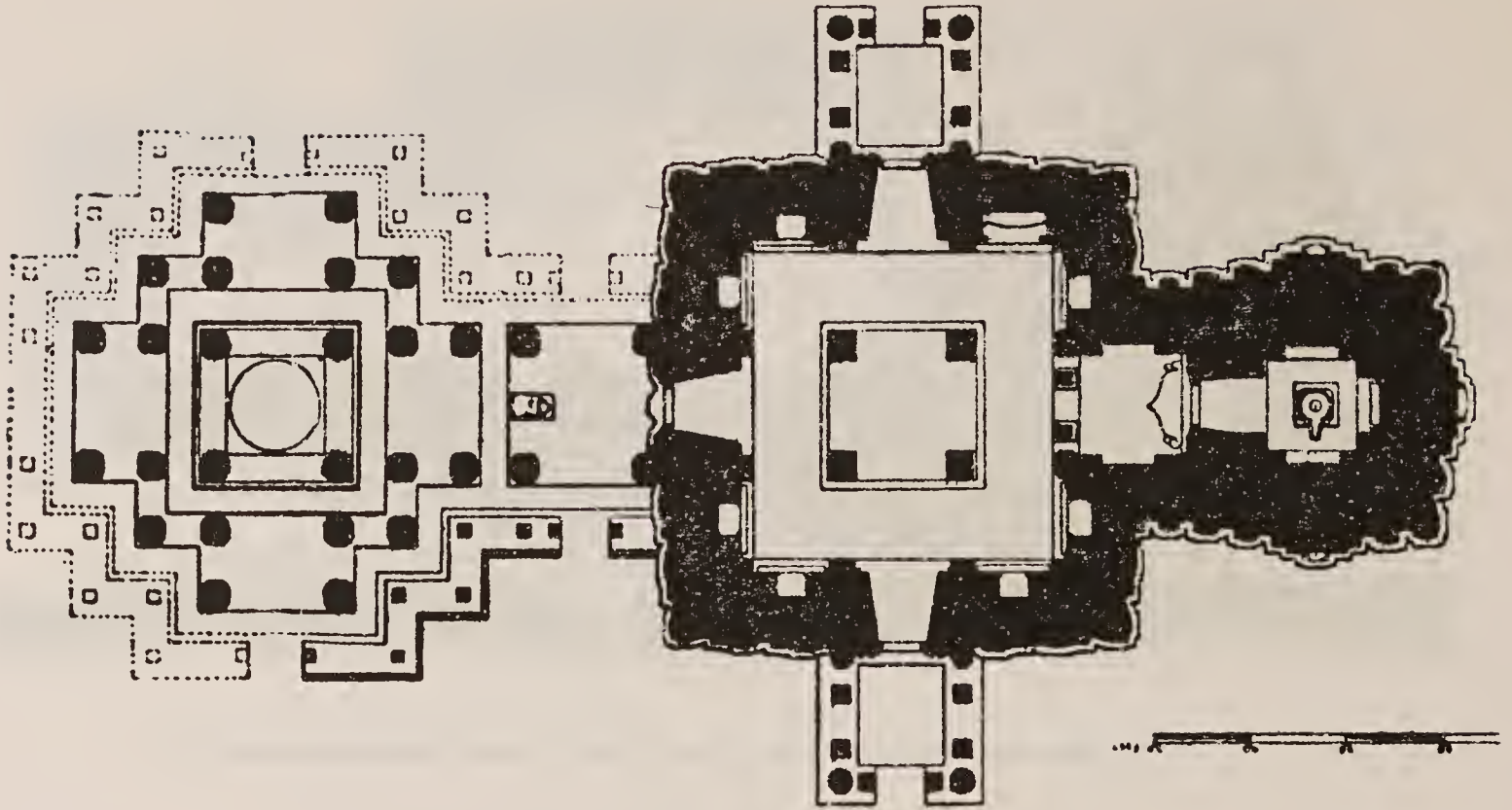
Fig. 46 Ittagi, Mahādeva temple: Plan
