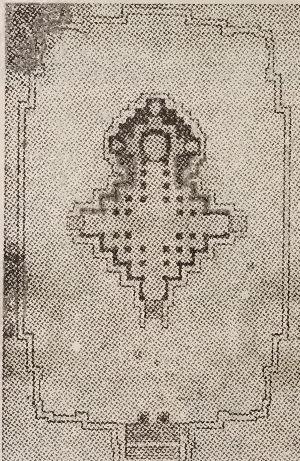
Fig. 20 Ghumli, Navalākhā temple: Plan
