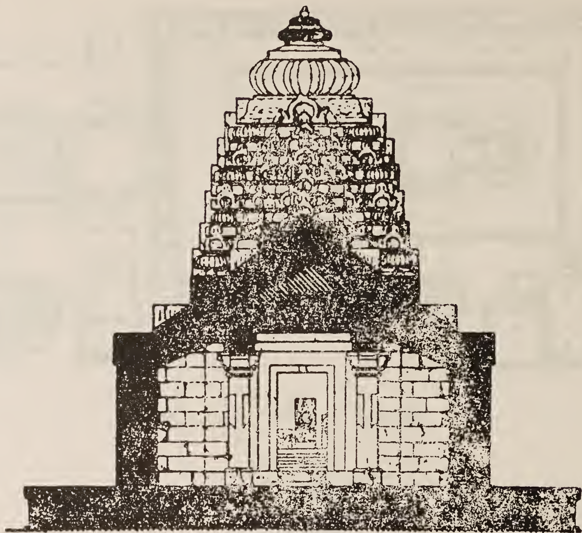
Fig. 15 Sutrapada, Sun Temple: Elevation
