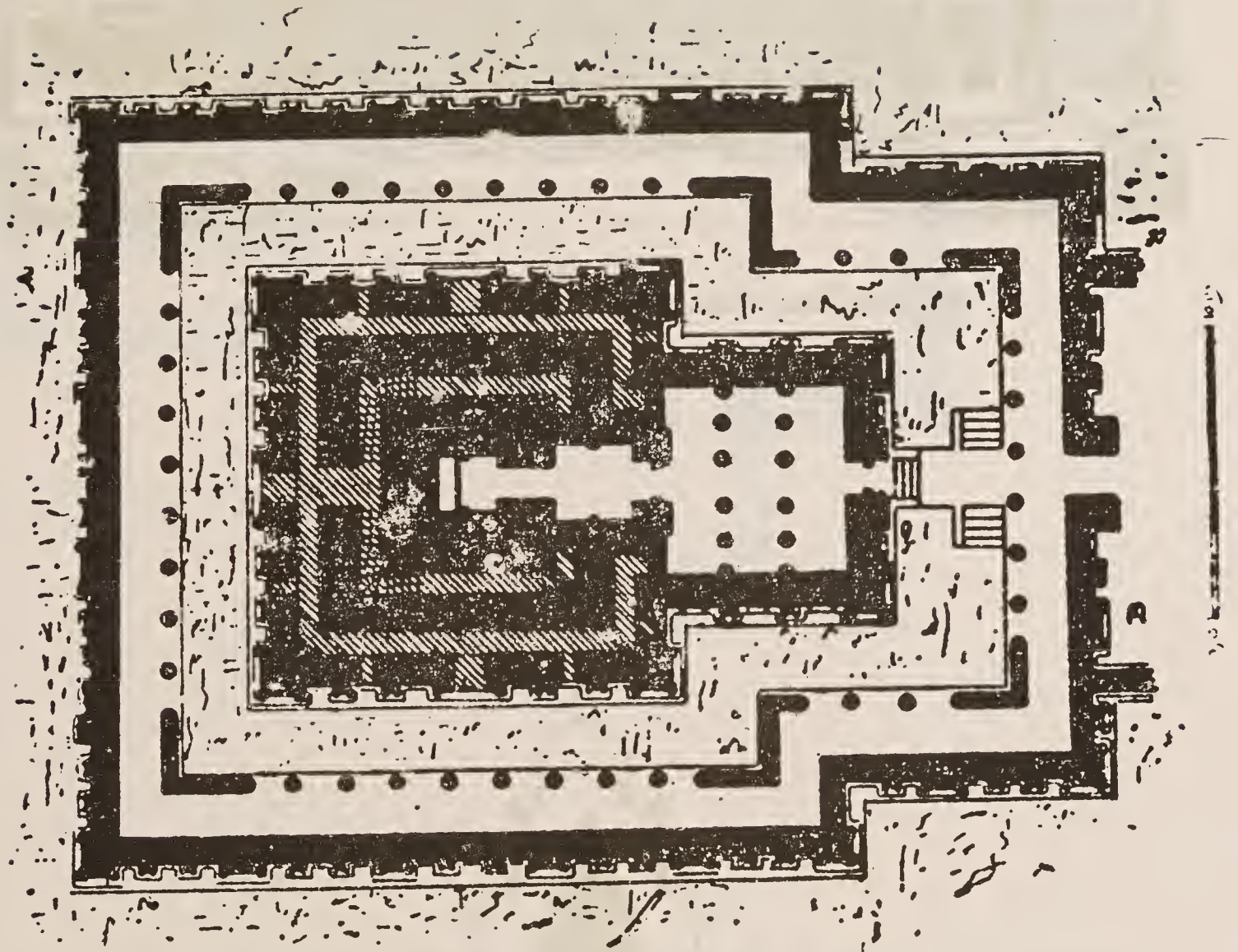
Fig. 34 Kāñchīpuram, Vaikuṇṭha Perumal temple: Plan
