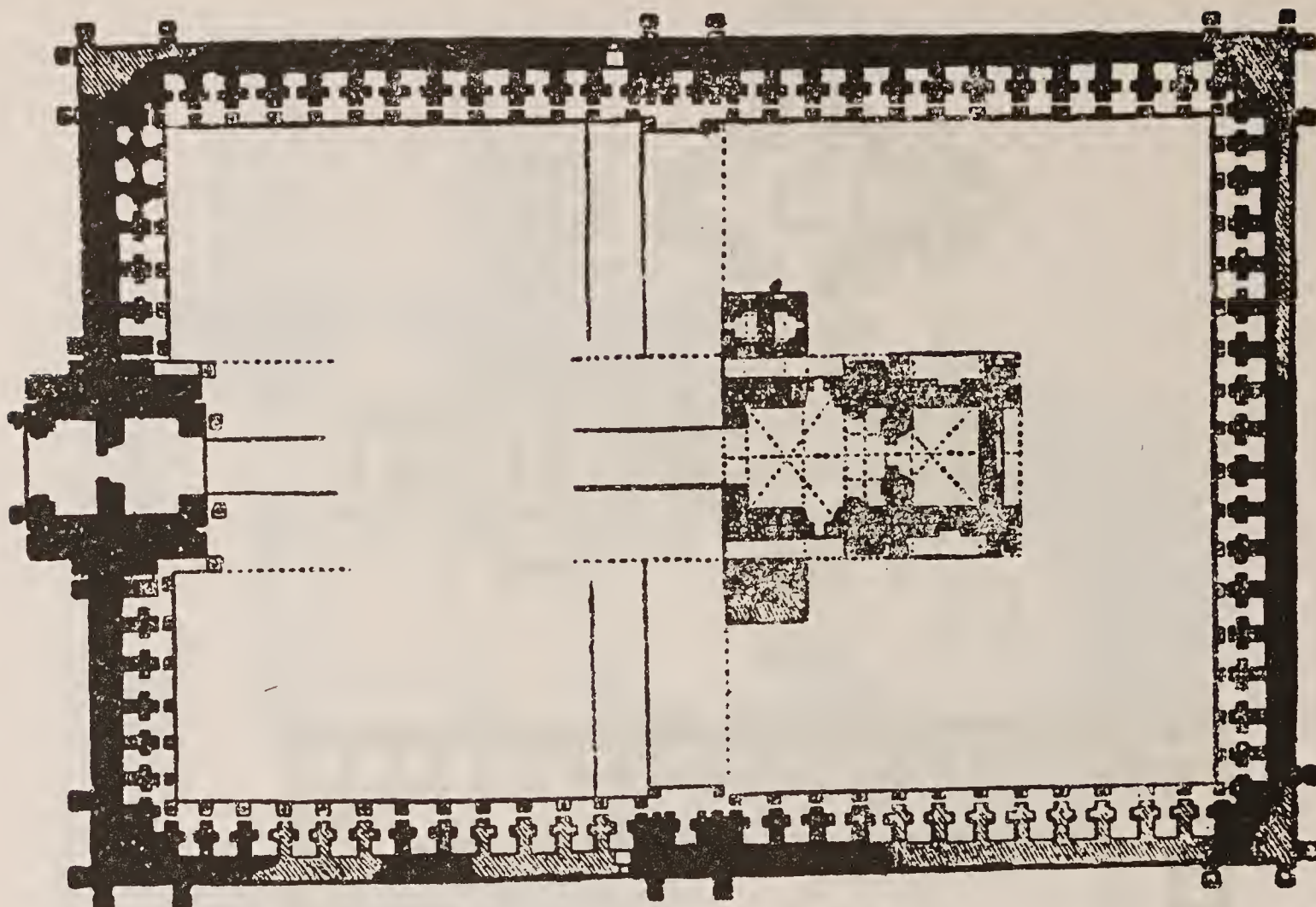
Fig. 54 Mārtand, Sun temple: Plan
