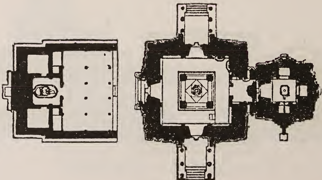
Fig. 47 Kuruvatti, Mallikārjuna temple: Plan
