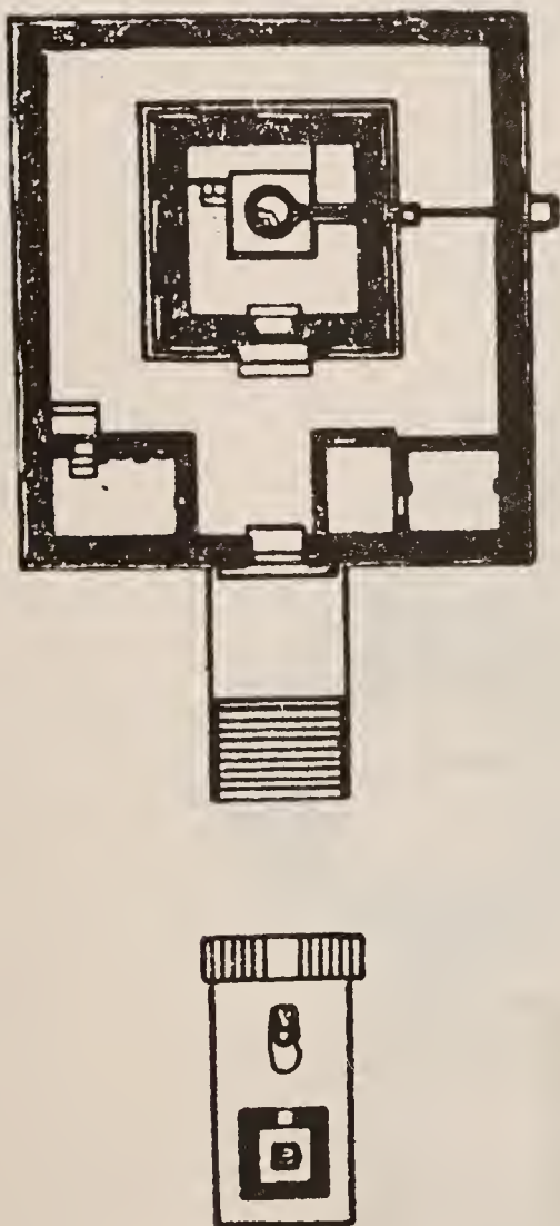
Fig. 13 Villesvara, Śiva temple: Plan
