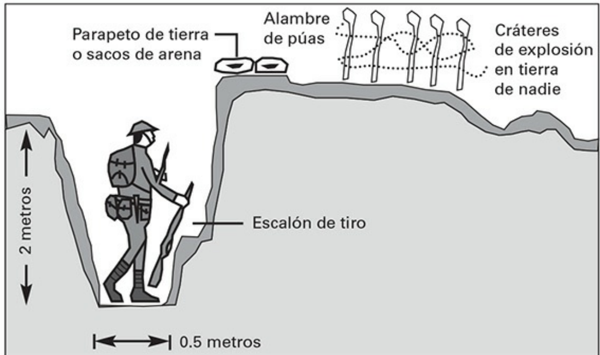
FIGURA II.1. Corte transversal de una trinchera
