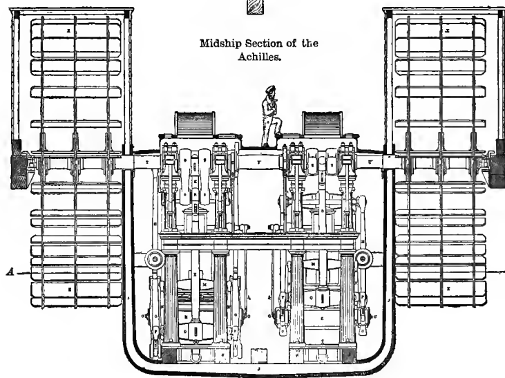
Engines and Paddles of H. M. S. Achilles.*
