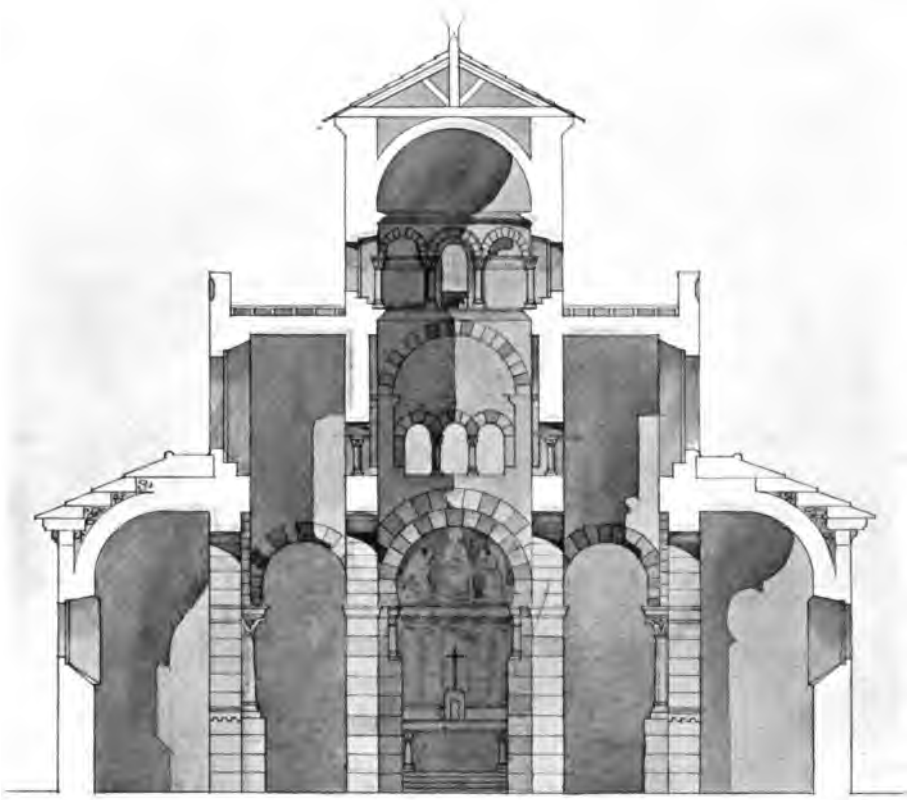
ILL. 89. — Section of Germigny-les-Prés
